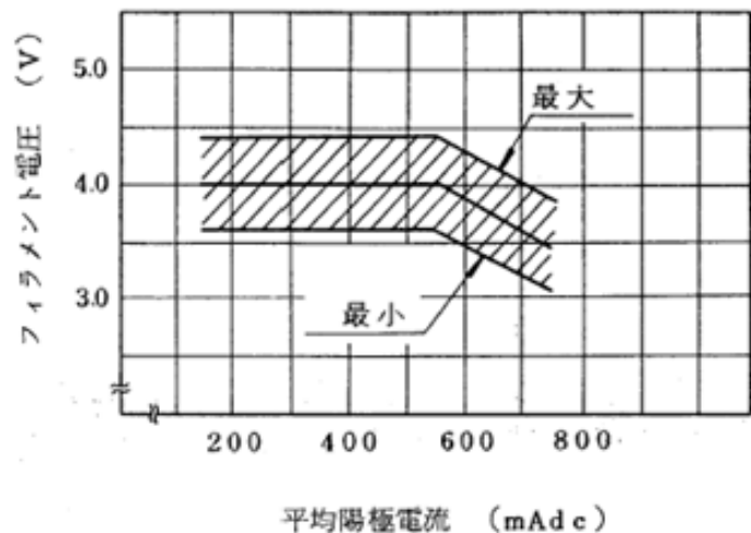
図1 フィラメント電圧低減カーブ
