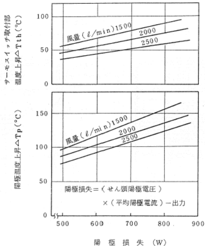
図 4 冷却特性
